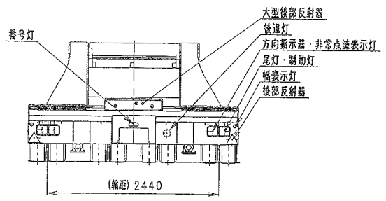
東急TD50J9T2S型 セミトレーラ外観四面図
